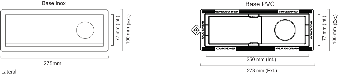
Vista Lateral
